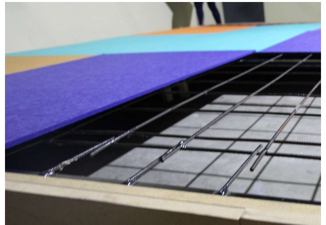
photo : détail du SlimPanel de 9mm sur le cadre métallique avec une espace d'air de 191mm
