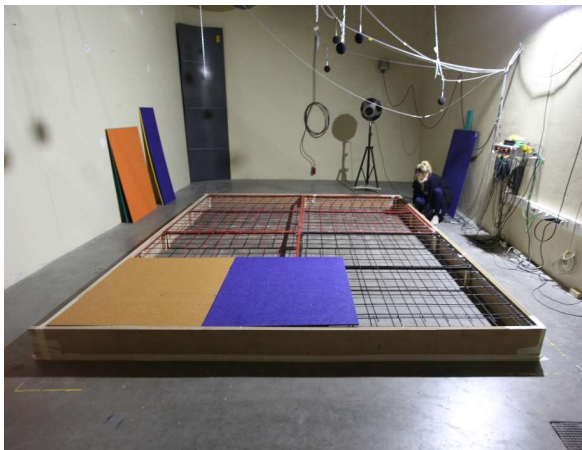
photo : détail du périmètre du spécimen d'essai
