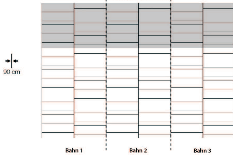
3 Verlegemöglichkeiten
